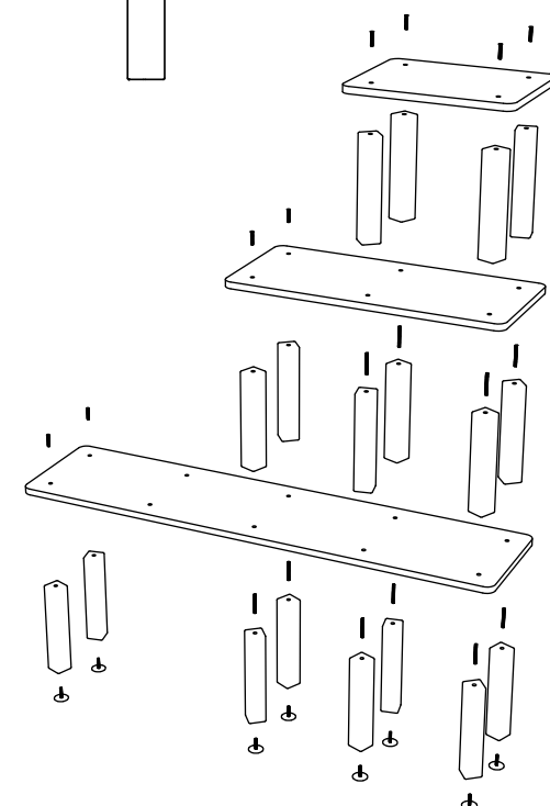
éclaté
