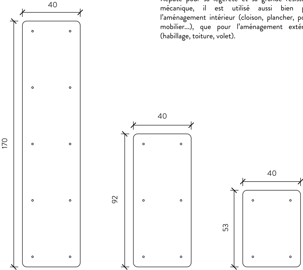
Vue du dessus, unité cm
