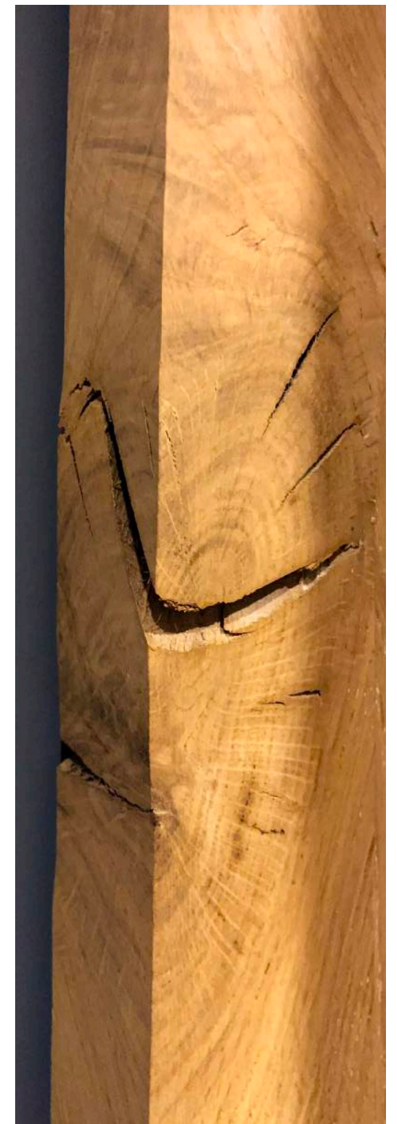
Bois comportant des défauts révalorisés dans le bâtiment (parement et châssis de porte)
