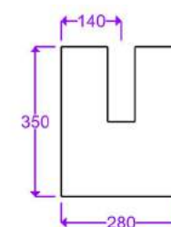
socle en granit D - percuteur
