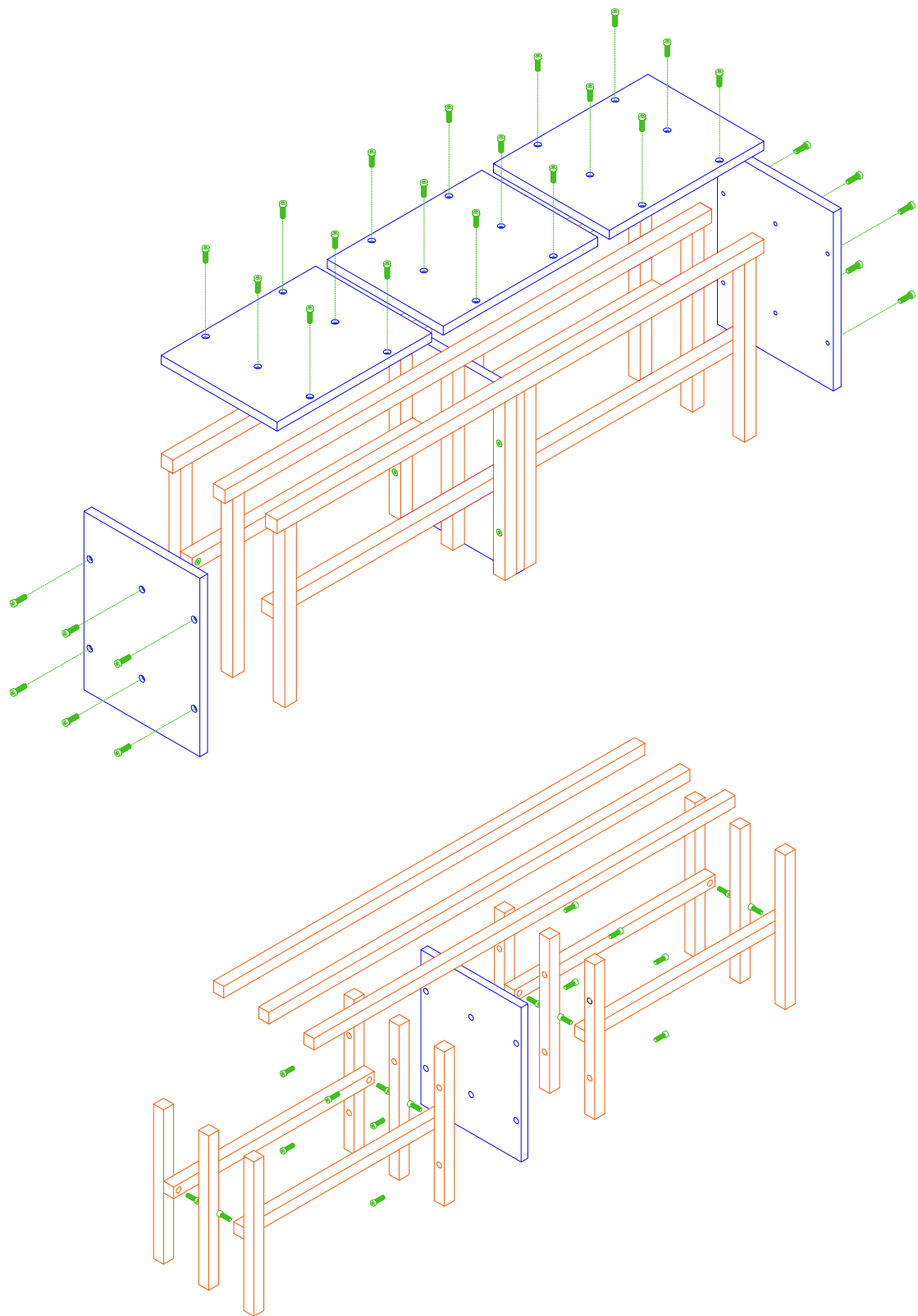
Principe d'assemblage sur le banc
